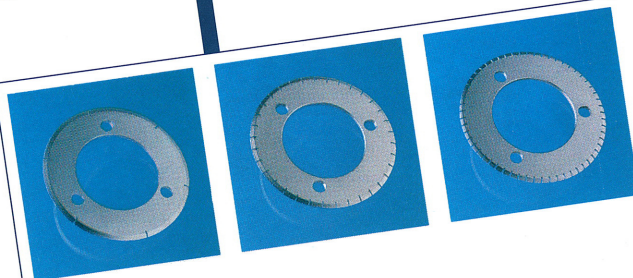
COLTELLO CIRCOLARE PERFORATORE Ø70,3X40X2 CON FORI DI FISSAGGIO NEI PASSI A RICHIESTA
